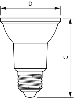
PAR20 120V 6W-50W 500lm 25D 3000K E26 D
